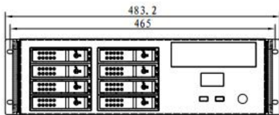
P向视图
